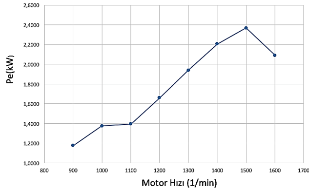
Grafik 1. Motor hızına bağlı olarak efektif güç değişimi (Graphic 1. Effective power change depending on engine speed)
