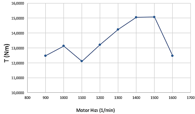
Grafik 2. Motor hızına bağlı olarak torkun değişimi (Graphic 2. Variation of torque depending on engine speed)
