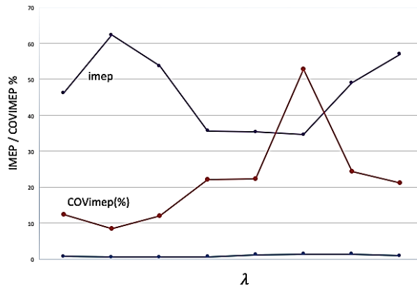
Grafik 13. Hava-yakıt denklik oranının ( \lambda ) bir fonksiyonu olarak IMEP ve COVimep (%)
