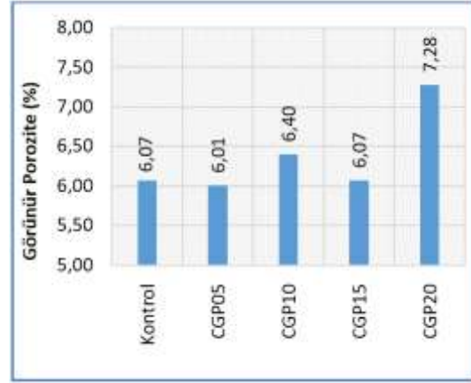
Şekil 3. Görünür Porozite (Figure 3. Visible Porosity)
