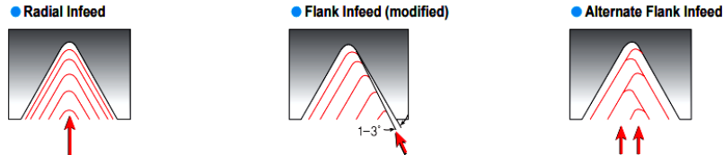
Şekil 1. Kademeli dış açma işlemi şekilleri (Figure 1. Gradual threading process figures)
