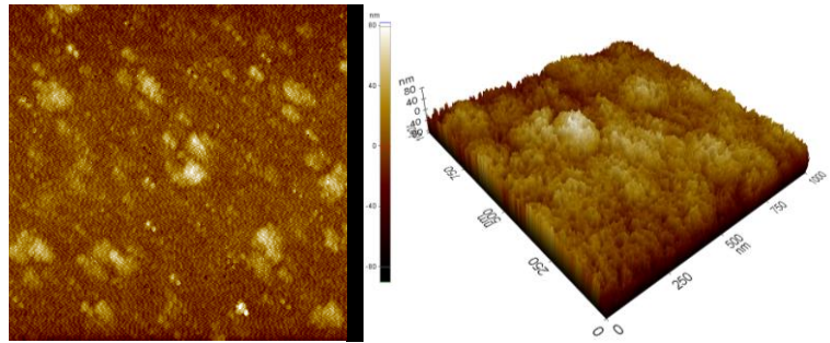
Şekil 5. %2 Zn katkılı CuO ince filminin 40\mu\text{m}\times 40\mu\text{m} 'deki 2 boyutlu ve 1\mu\text{m}\times 1\mu\text{m} 'daki 3 boyutlu görüntüsü.
