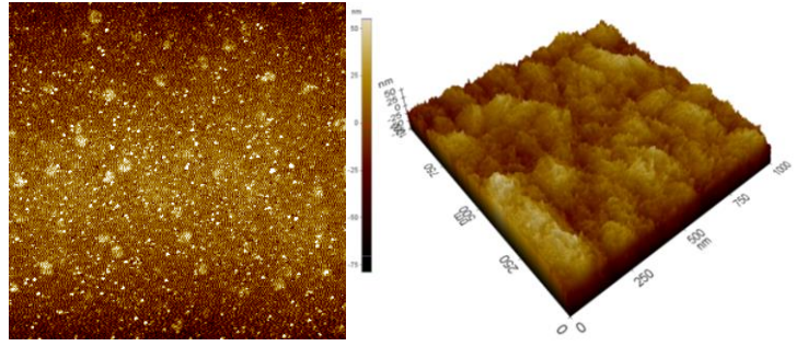
Şekil 4. %0.5 Zn katkılı CuO ince filminin 40\mu\text{m}\times 40\mu\text{m} daki 2 boyutlu ve 1\mu\text{m}\times 1\mu\text{m} daki 3 boyutlu görüntüsü.
